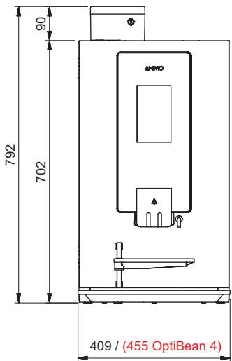
OPTIBEAN VOORKANT
