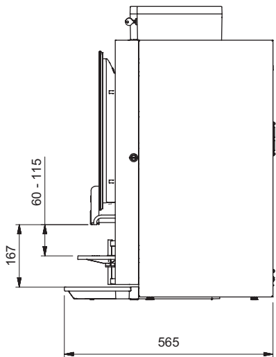
ZIJAANZICHT RECHTS
