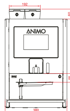
VOORZIJD
